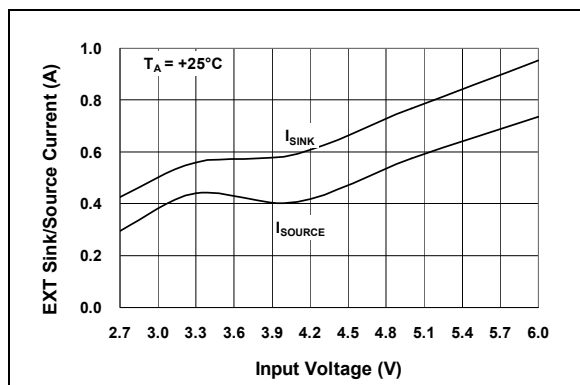
图 2-7: EXT 灌电流和拉电流—输入电压曲线
