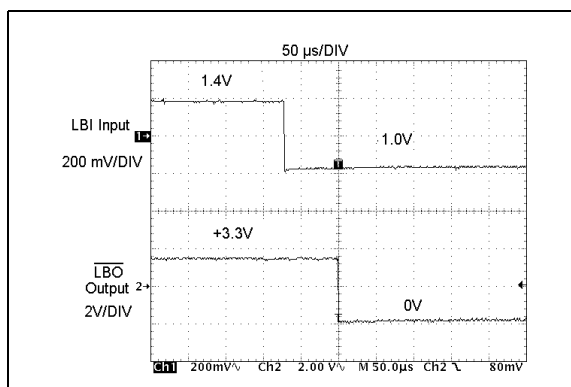
图 2-24: \overline{LBO} 输出时序图
