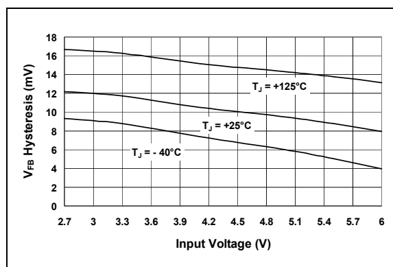
图 2-11: 反馈电压额定迟滞—输入电压曲线
