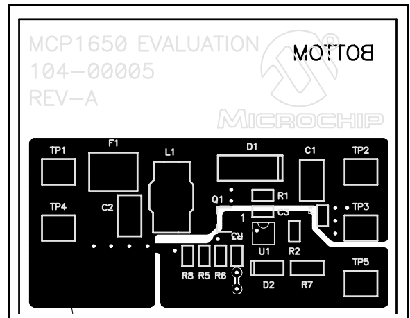
图 6-3: 底层走线
