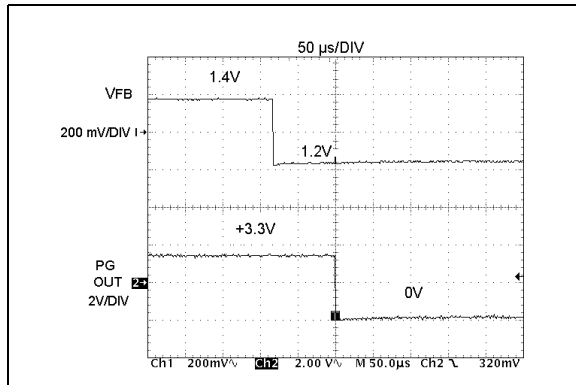
图 2-27: PG 时序图
