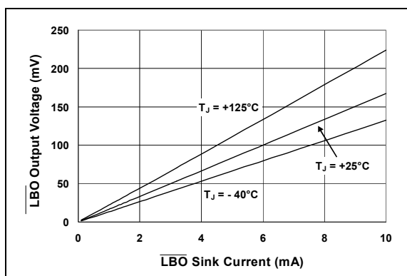
图 2-23: \overline{LBO} 输出电压— \overline{LBO} 灌电流曲线
