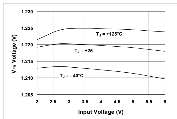
图 2-10: 反馈电压—输入电压曲线
