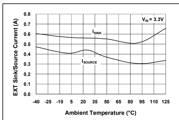
图 2-8: EXT 灌电流和拉电流—环境温度曲线
