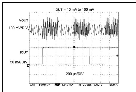
图 2-12: 动态负载响应
