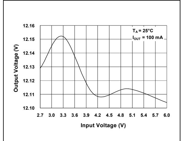
图 2-18: 输出电压—输入电压曲线 (线路稳定)
