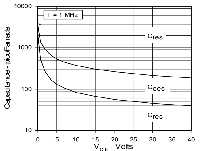
Fig. 16. Capacitance
