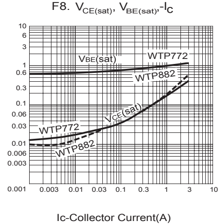
V_{CE(sat)}, V_{BE(sat)}-I_C
