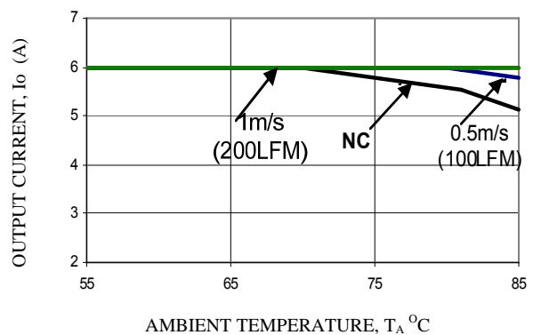
V_o = 5.0V
