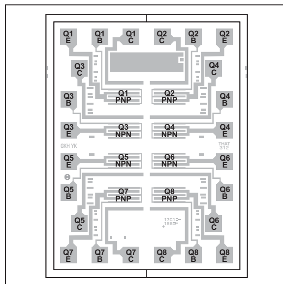
Fig 4. 380 Die layout
