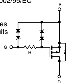
P-Channel MOSFET
