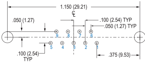
9 PIN MWDM-9PBS
