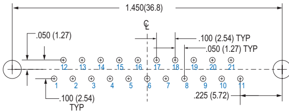
21 SOCKET MWDM-21SBS
