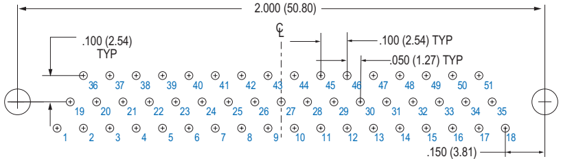
51 SOCKET MWDM-51SBS
