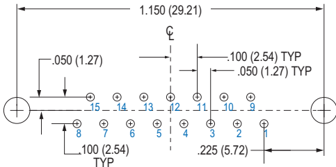
15 PIN MWDM-15PBS
