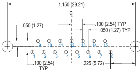
15 SOCKET MWDM-15SBS
