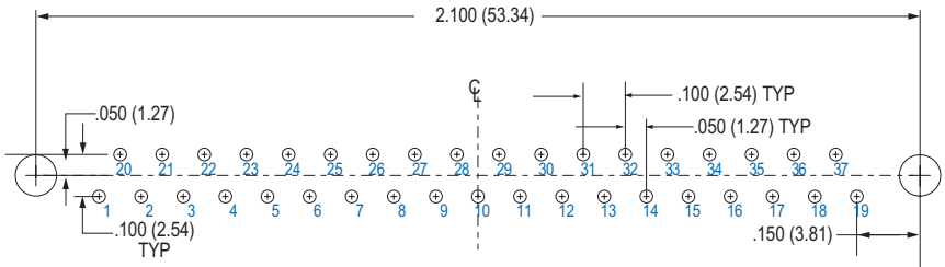
37 SOCKET MWDM-37SBS
