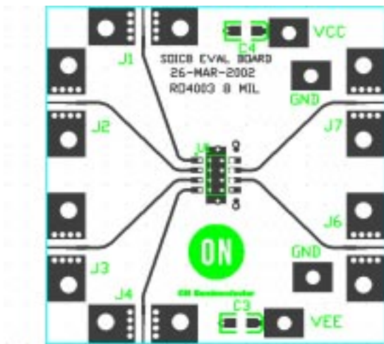
Top Layer
