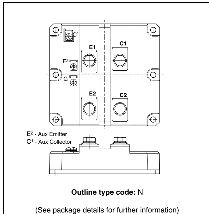
Fig. 2 Module outline
