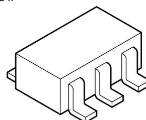
SSOP5-P-0.95
