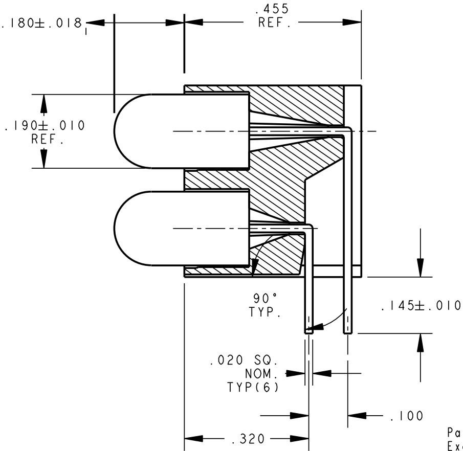
SECTION A-A
