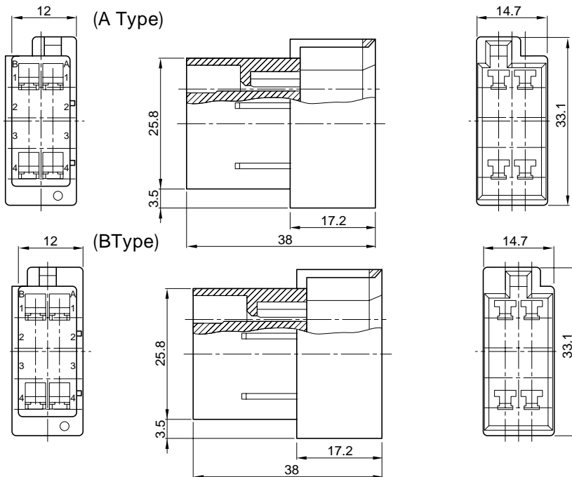
8P Plug 8Pプラグ CSC 3008-02□□
