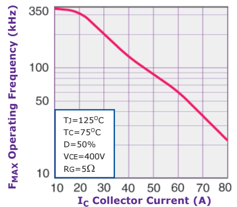
1200 Volt Size 6 - APT35GP120B2D2
