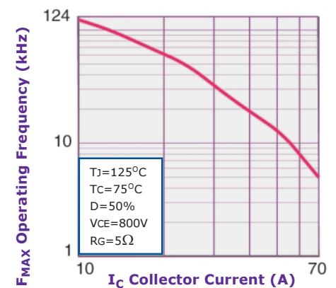
1200 Volt Size 6 - APT35GP120B2D2
