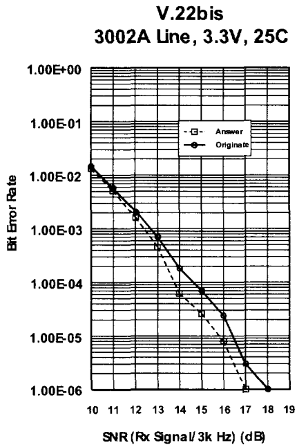
BER VS SNR
