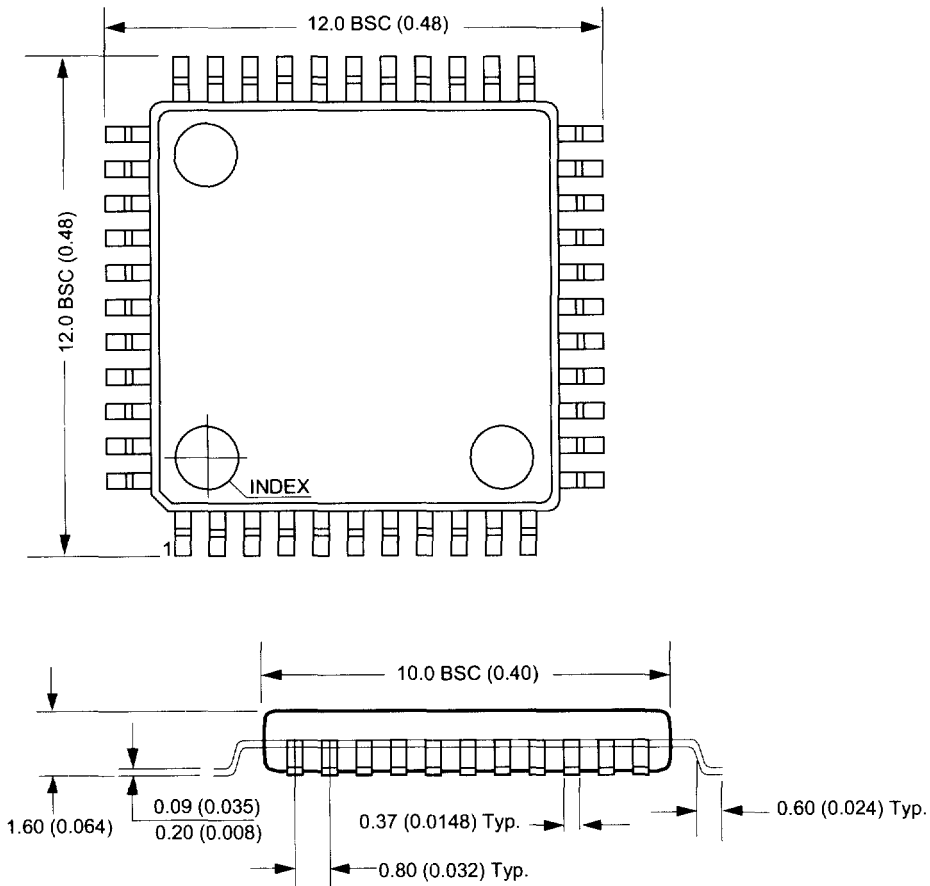
44-Pin TQFP (JEDEC LQFP)
