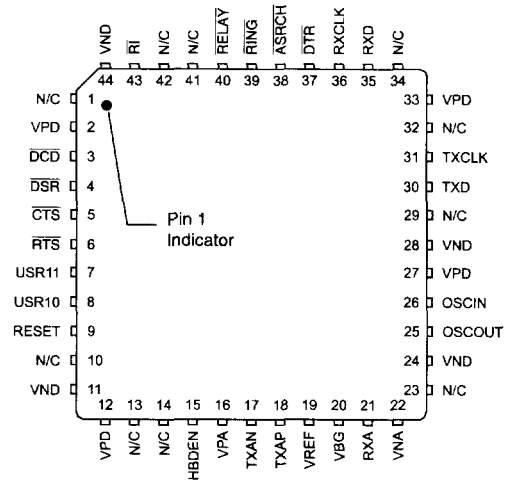
44-Pin TQFP 73M2901-IGT/3
