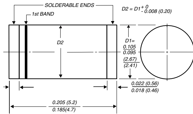
DO-213AB (GL41)
