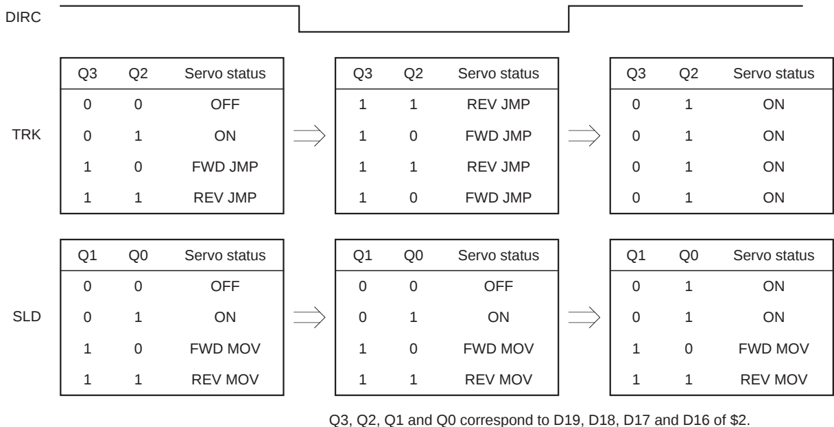
Fig. 5-22.
