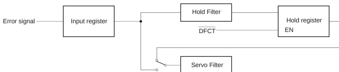
Fig. 5-13.
