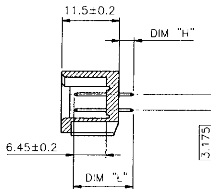
SECTION V-V
