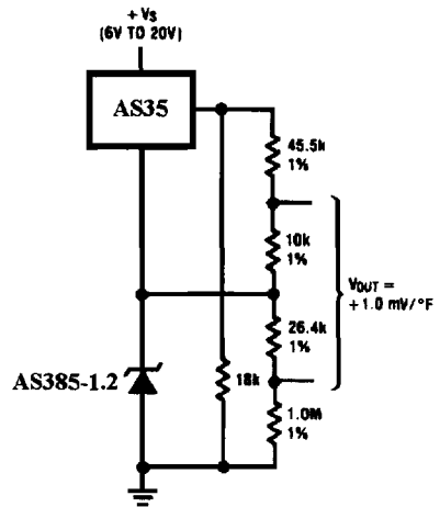
Fahrenheit Thermometer
