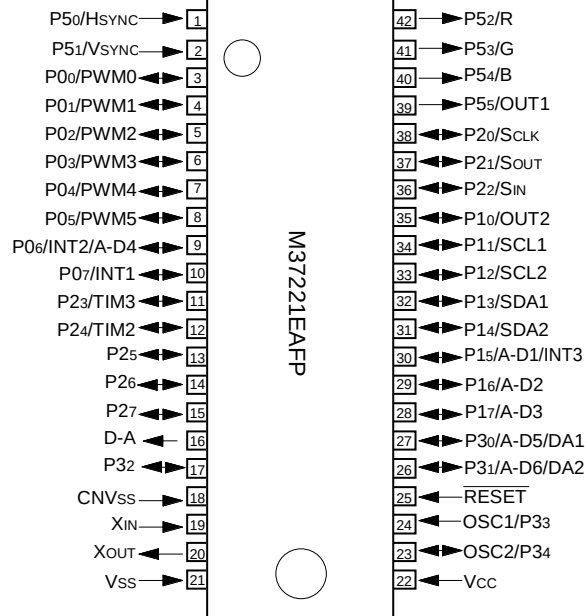
Outline 42P2R-A/E
