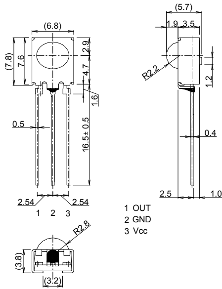
NJL31V000A-M UNIT:mm
