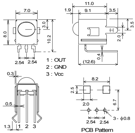
NJL33H000A UNIT:mm
