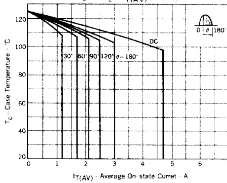
Fig. 11 T_c - I_T(AV) RATING
