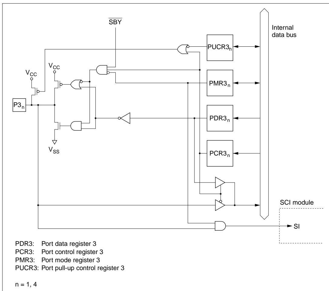
Figure C.3 (d) Port 3 Block Diagram (Pins P3_4 and P3_1 )
