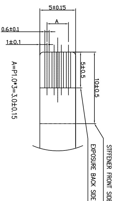
Detail "AA"(Scale=6/1)
