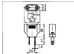
AC ADAPTER ACアダプタ
