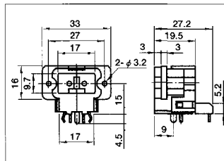
AC INLET (WITH SWITCH) ACインレット (スイッチ付)
