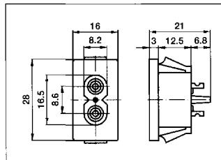
AC INLET (IEC TYPE) ACインレット (IECタイプ)
