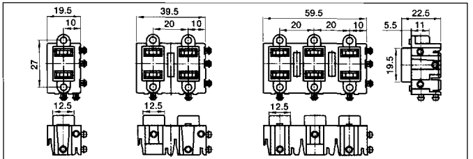
AC OUTLET ACアウトレット
