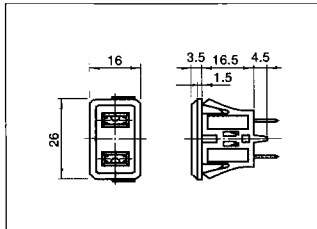
AC OUTLET (FASTON TYPE) ACアウトレット (ファストン端子対応タイプ)
