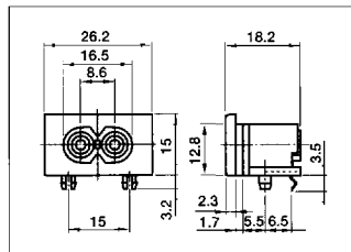
AC INLET (DIP TYPE) ACインレット (DIPタイプ)
