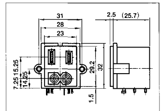
AC INLET/OUTLET ACインレット・アウトレット一体タイプ
