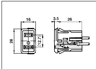
AC OUTLET (CRIMP TYPE) ACアウトレット (圧着タイプ)
