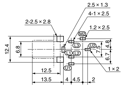
JPJ5412 JPJ5112
