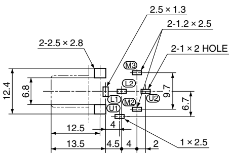
JPJ5421 JPJ5121
