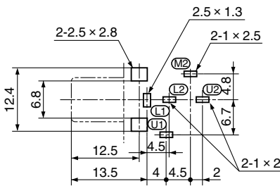
JPJ5411 JPJ5111
