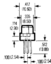
Wire Wrap
