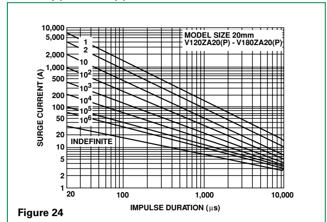
V120ZA20(P) - V180ZA20(P)
