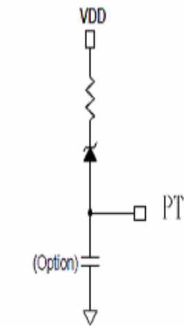
V_{DD} OVP : V_{DD} > V_R + V_Z + 4V VDD OVP Only
