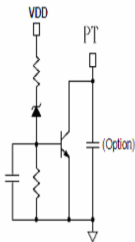
VDD OVP
