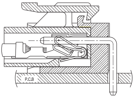
PCB ASS'Y
