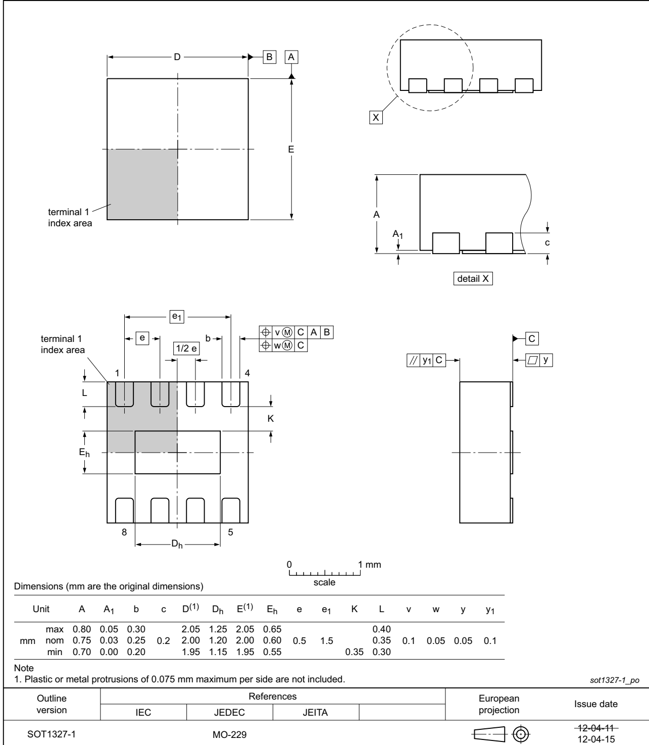
Fig 16. Package outline SOT1327-1 (HWSON8)
