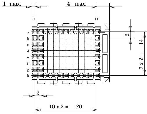
Bestückungsplan - contact layout
