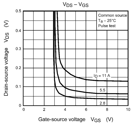
Fig. 8.4 V_{DS} - V_{GS}
