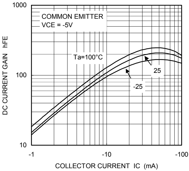
hFE - IC
