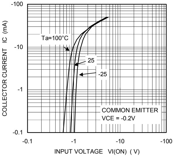
IC - VI(ON)
