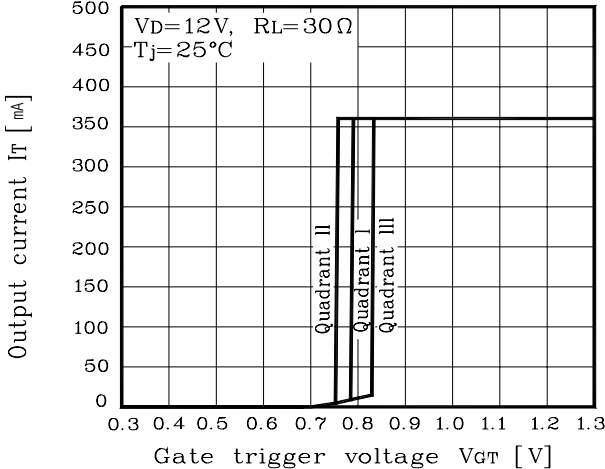
Fig. 8 I_T - V_{GT}
