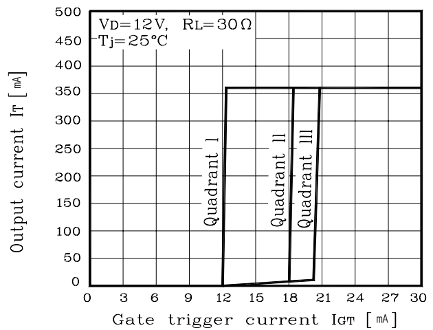
Fig. 6 I_T - I_{GT}
