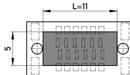
Leiterplatten-Layout Rückseite PCB-Layout Back Side
