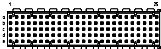
Bestückungsplan - contact layout
