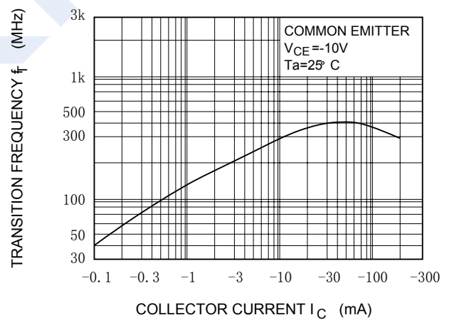
f_T - I_C
