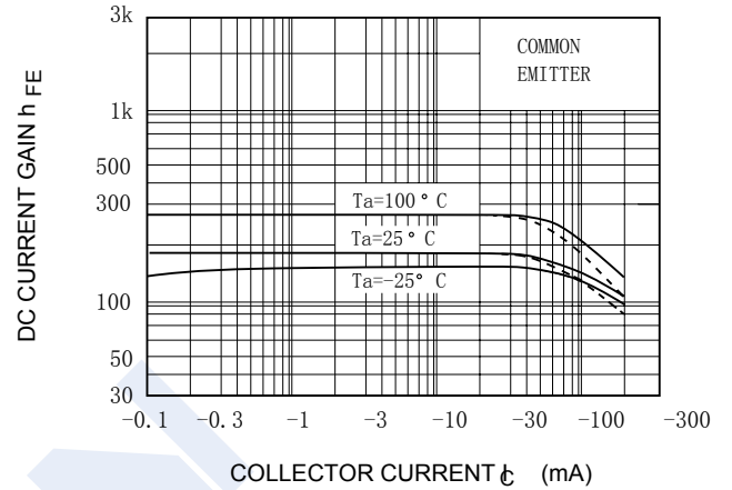
h_{FE} - I_C
