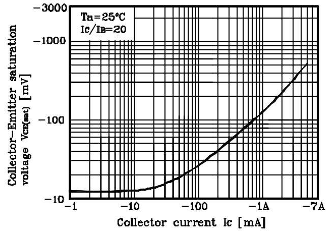
Fig. 4 V_{CE(sat)} - I_c
