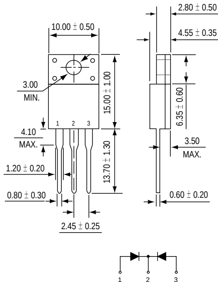
ITO-220AB
