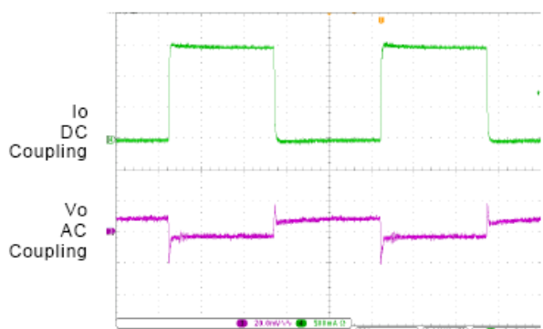
12. Load Transient
