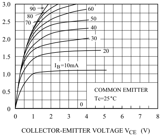
I_C - V_{CE}
