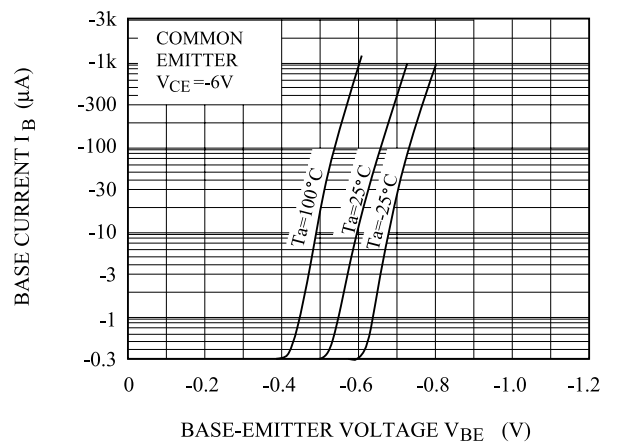
I_B - V_{BE}
