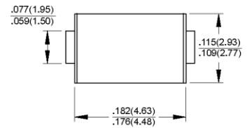
DO-214AC (SMAJ)
