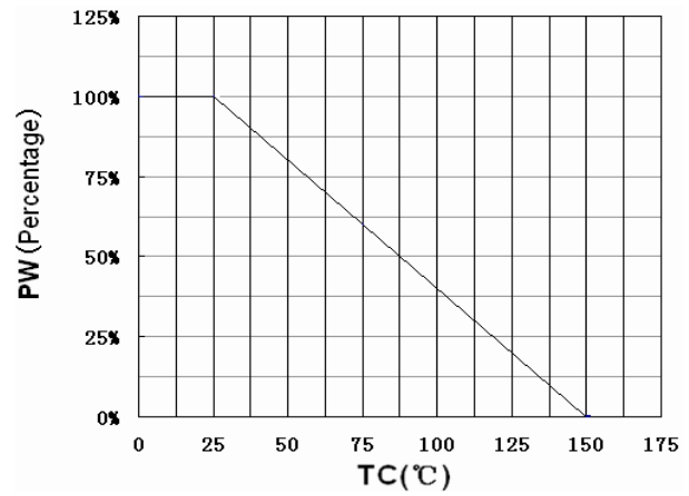
P_C - T_C
