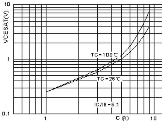
V_{CE(sat)} - I_C
