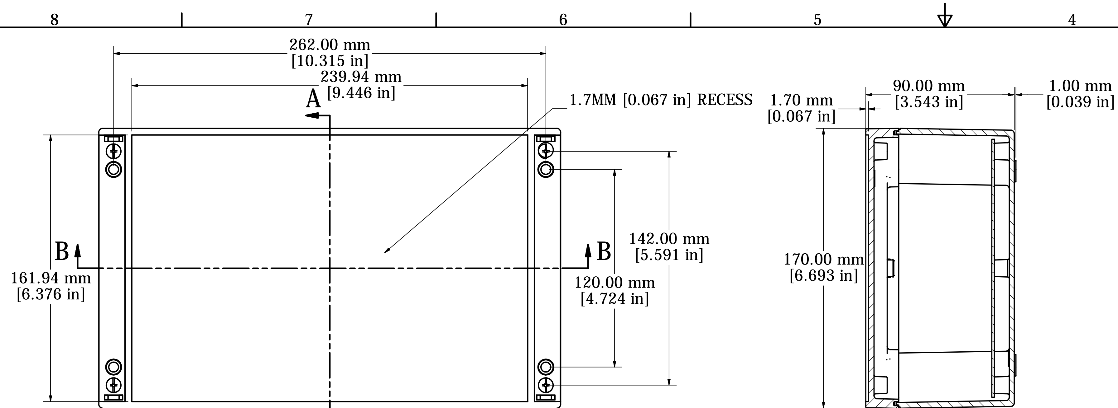
SECTION A-A
