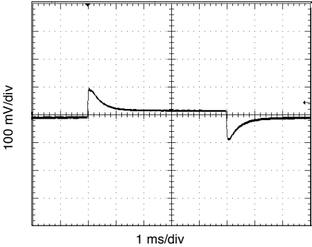
Load 50 - 100 - 50%, 28 Vin
