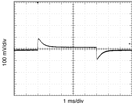
Load 50 - 100 - 50%, 50 Vin
